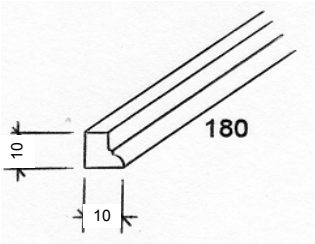
Bandeau du socle cheminée réf : 60028
