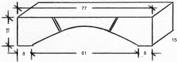
Cintre de cheminée réf : 60200
