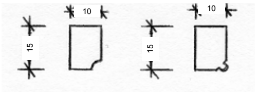
Coin de hotte moyen 15x10x17 réf : 60062
