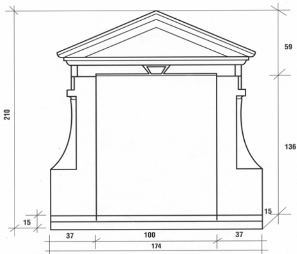
Lucarne Luc6 Réf : 81360
