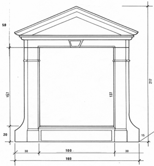
Lucarne Luc5 Réf : 81359
