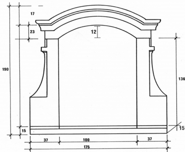
Lucarne Luc3 Réf : 81357
