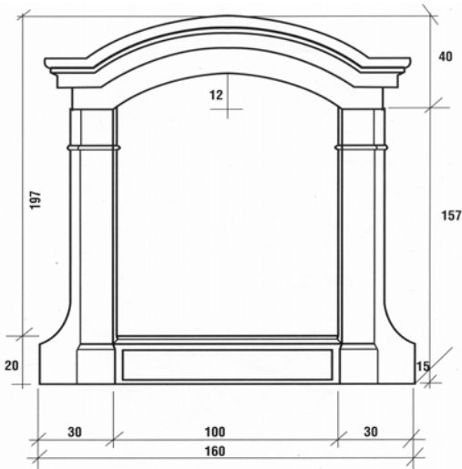
Lucarne Luc6 Réf : 81360
