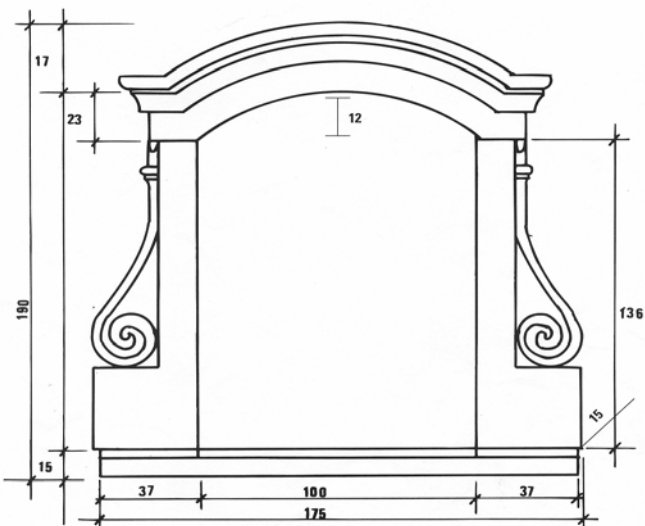
Lucarne Luc3 Réf : 81357
