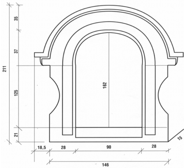
Lucarne Luc2 Réf : 81356
